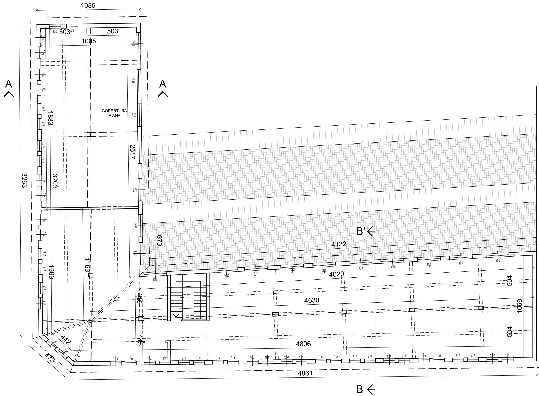
PIANTA PIANO SOTTOTETTO
