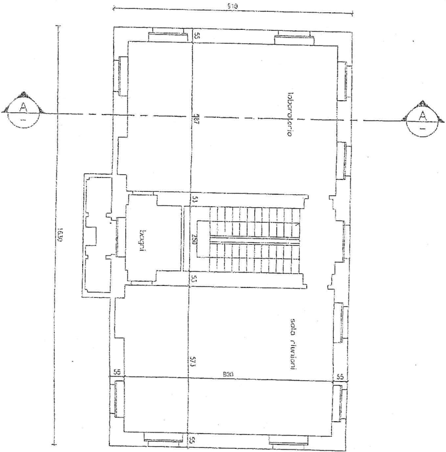
PRIMO PIANO - quota (+4,80m)
